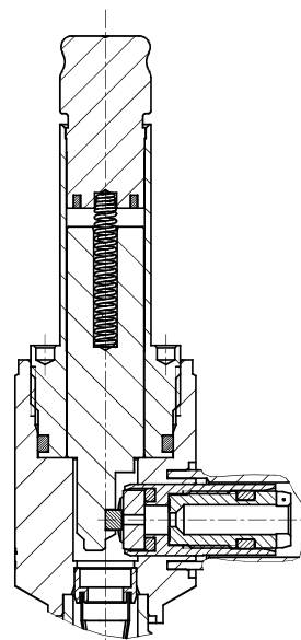
EX2 разрез (не по оси)
