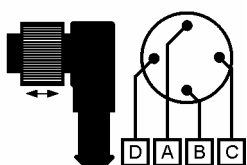
EX5-N/L/C... Кабель с разъемом в сборе
